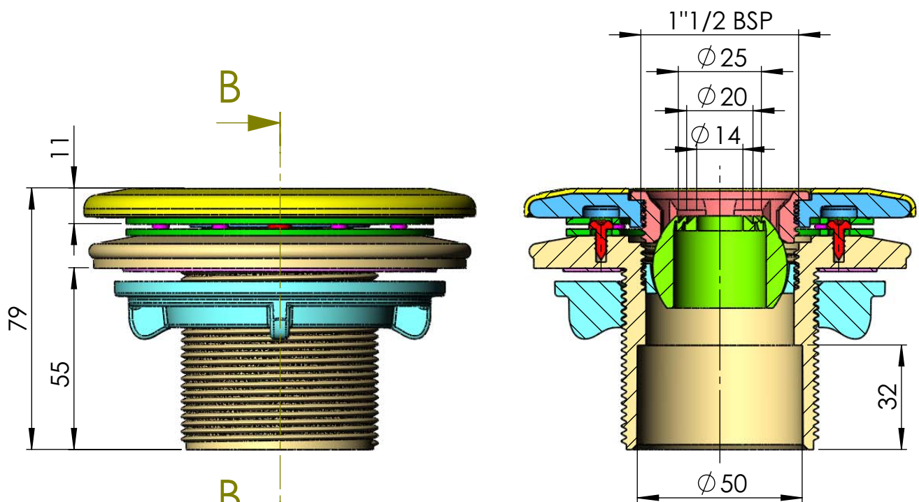
SECCIÓN B-B
